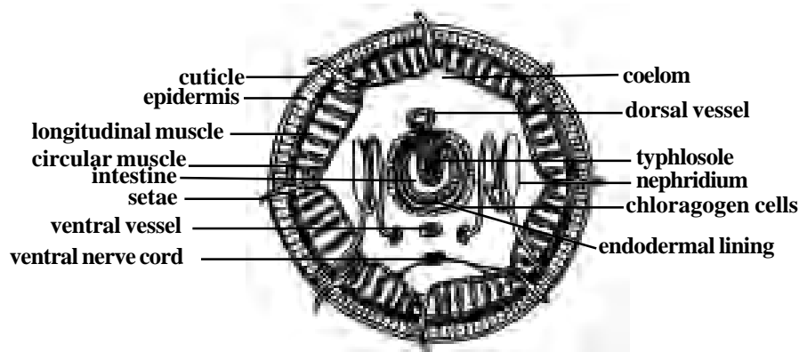
Fig. 1.3.3. Earthworm-T.S.
