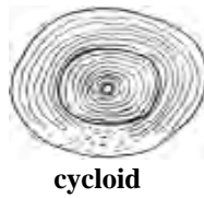
Fig. 1.2.22 Scales
