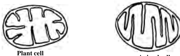
Fig.2.2.4. Mitochondria
