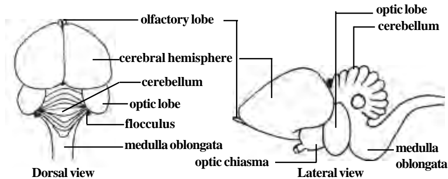
Fig. 1.3.19. Pigeon - Brain
