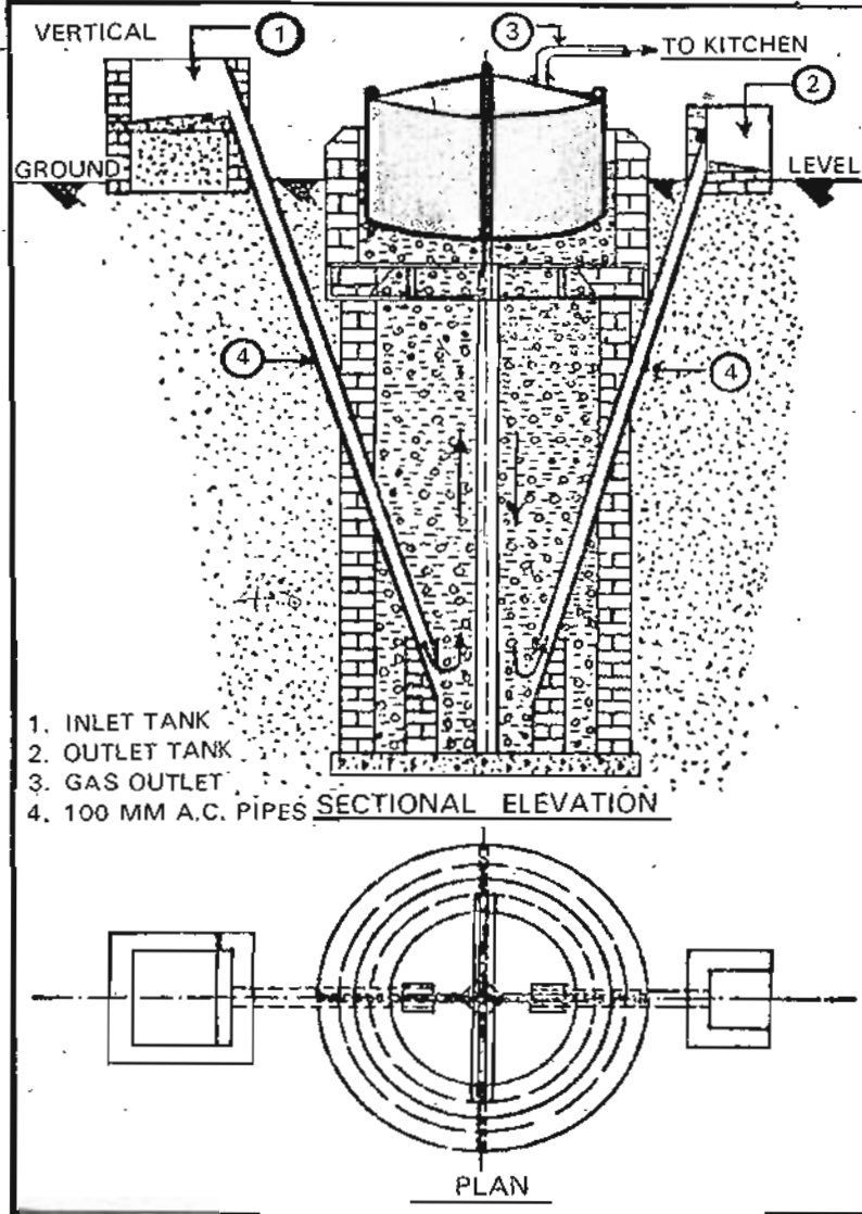
Fig. 19. R. V. I. C. design
