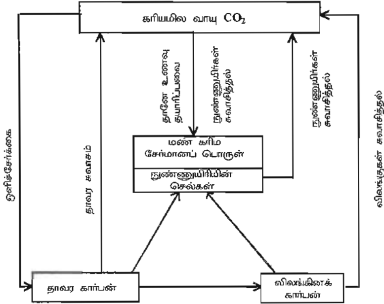
6-3 காற்பன் சுழற்சி
